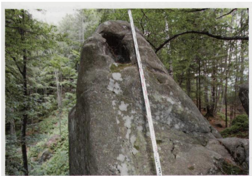
Лесівські камені. Скеля з врубом.
