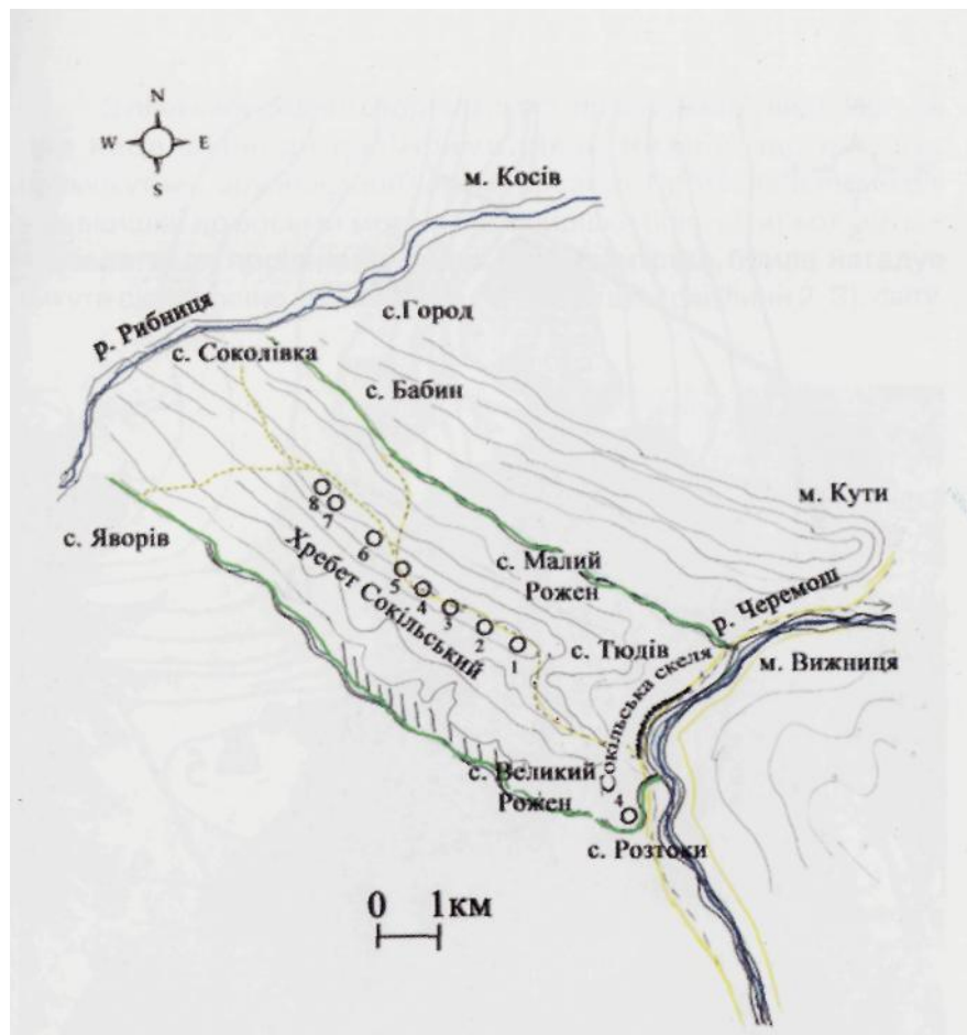
Малюнок 1. Сокільський хребет. Скельні комплекси
